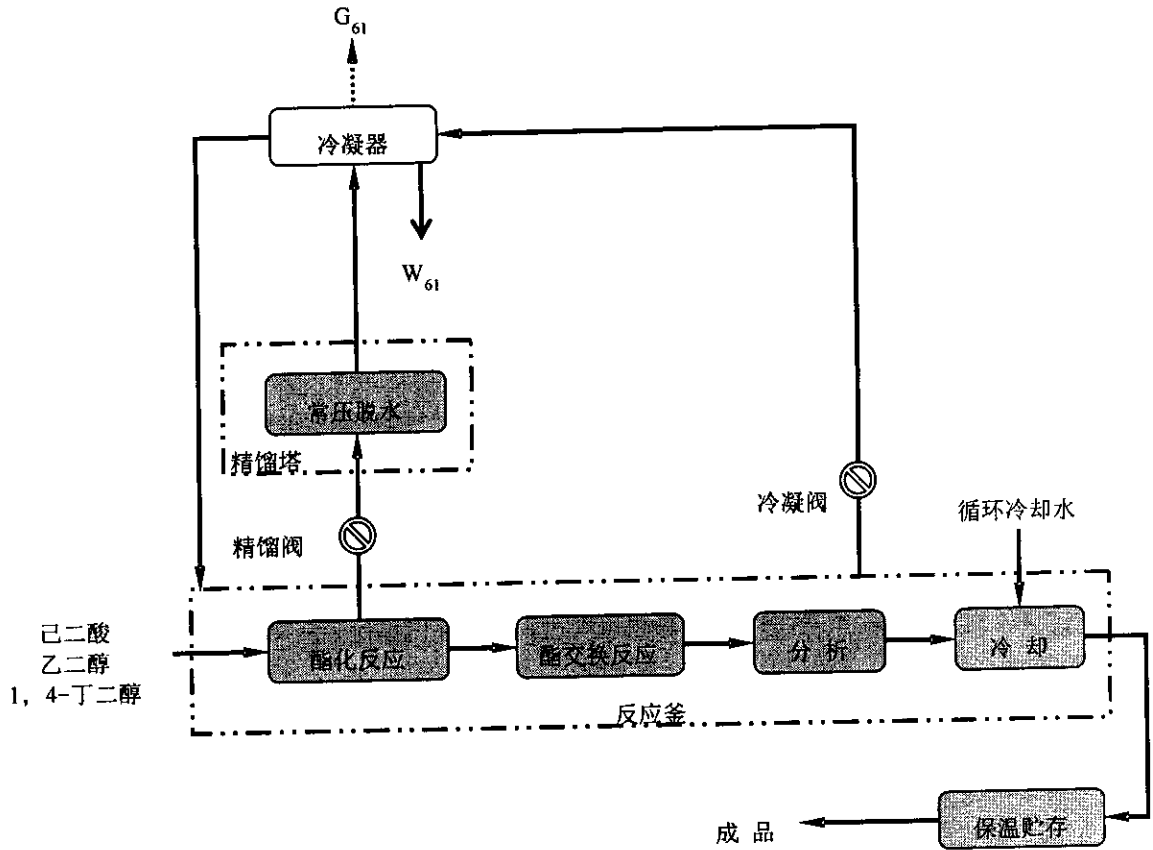
聚酯多元醇工艺流程
